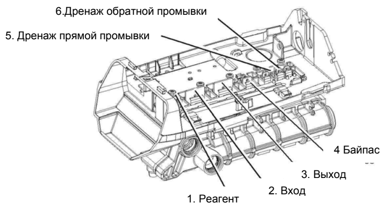
Рис. 15. Управляющий клапан Performa (263, 268)
