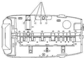
Монтажные отверстия
